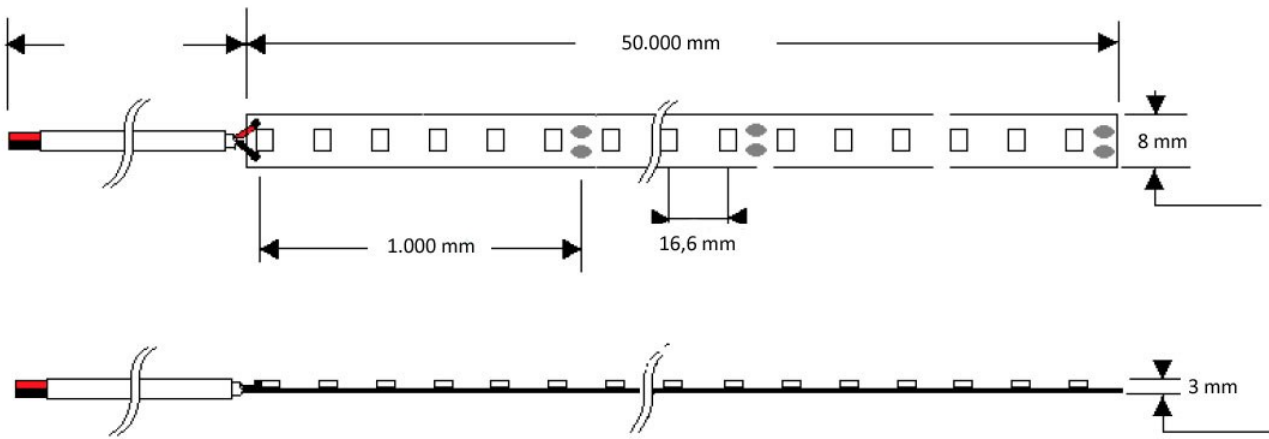
Målskitse for 230V Led strip 60 Led/m uden silikone indstøbningen
